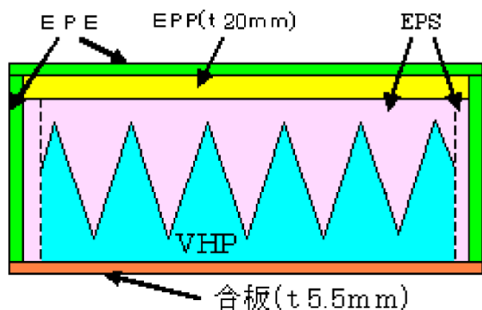
図1 ECCOSORB® VHP-FLの構造
